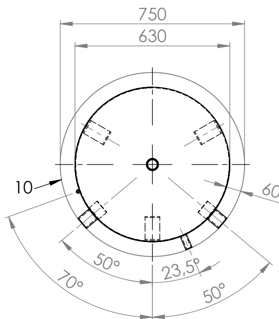
Pufferspeicher 500l 195.0550
